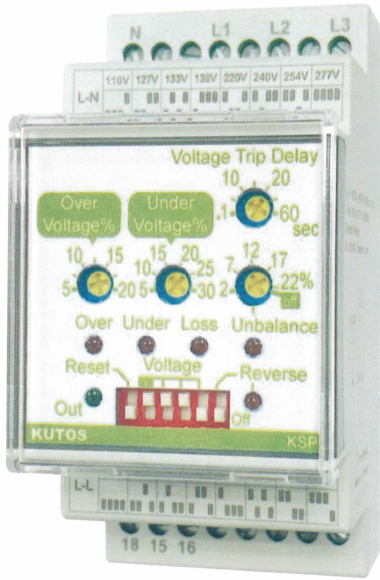
高低壓欠逆相三相不平衡保護 (圖一)
