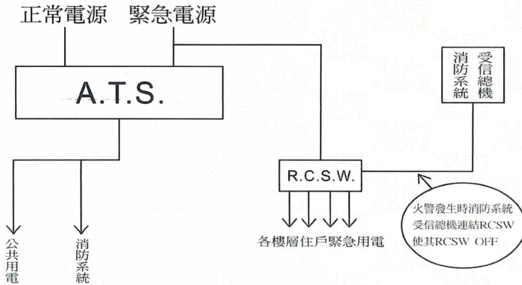
R. C. S. W. 系統說明示意圖
